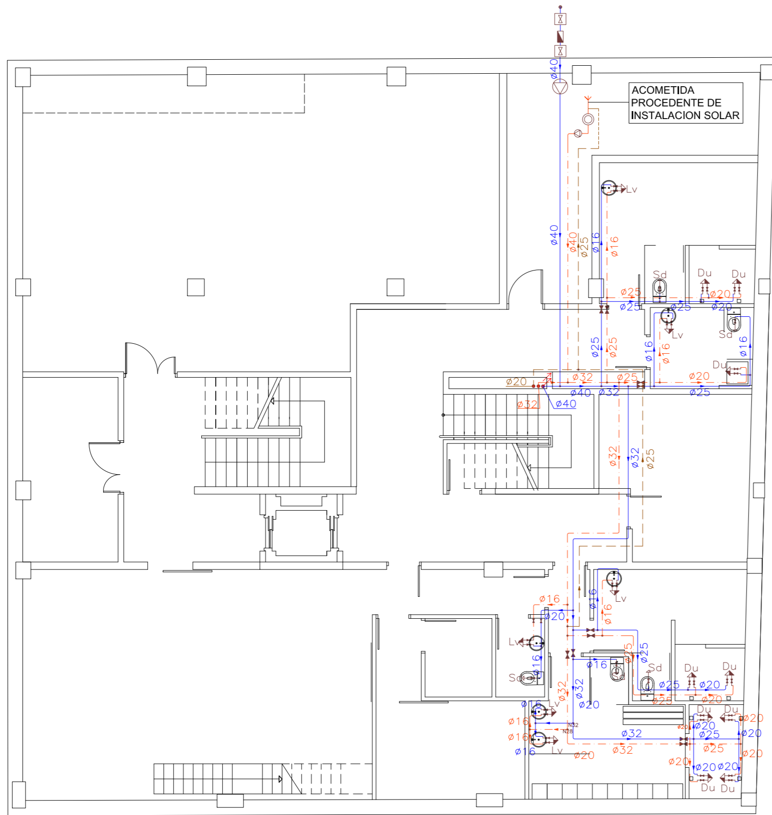
PLANTA SÓTANO
