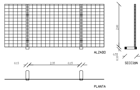
DETALLE DE VALLA DE PROTECCIÓN PERIMETRAL
