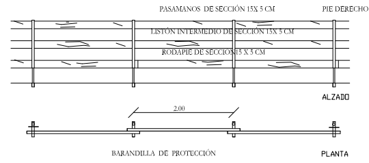
DETALLE DE BARANDILLA DE PROTECCIÓN
