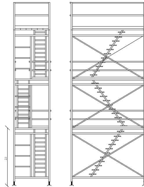
ESCALERAS DE ACCESO A L VACIADO, SÓTANOS 2 Y 1
